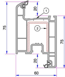
1. Dar Kapı Kanat Profili P.A.900.2107.600.0.BC.01 2. Destek Sacı (42x30x42) 1,2mm 34022-12023 1,5mm 34022-15023 2,0mm 34022-20023
