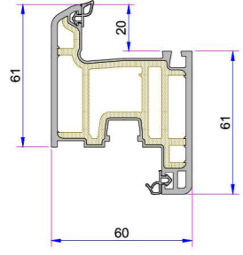
Penwood 760 Kanat Profili P.A.632.2000.600.2.BC.01
