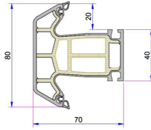
Penwood 760 Orta Kayıt Profili P.A.706.3000.600.2.BC.01
