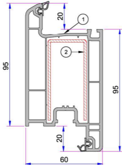
1. Kapı Kanat Profili P.A.632.2100.600.0.BC.01 2. Destek Sacı (62x30x62) 1,2mm 34022-12029 1,5mm 34022-15029 2,0mm 34022-20029
