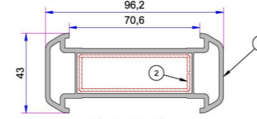
1. Kalın Bağ Profili P.A.070.5000.600.0.00.19 2. Destek Sacı (20x60) 1,2mm - 34022 - 12106 1,5mm - 34022 - 15106 2 mm - 34022 - 20106
