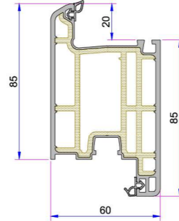
Penwood 760 Kapı Kanat Profili P.A.632.2100.600.2.BC.01
