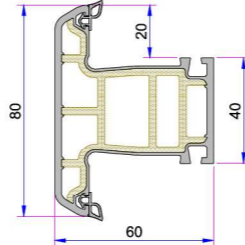
Penwood 760 Orta Kayıt Profili P.A.706.3000.600.2.BC.01
