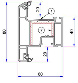
1. Dışa Açılım Kanat Profili P.A.632.2014.600.0.BC.01 2. Destek Sacı (30x30x18) 1,2mm 34022-12022 1,5mm 34022-15022 2,0mm 34022-20022
