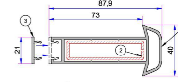
1. Ünlversal Kalın Bağ Profili P.A.058.5000.600.0.00.19 2. Destek Sacı (15x60) 1,2mm - 34022 - 12123 1,5mm - 34022 - 15123 2 mm - 34022 - 20123 3. Ünlversal Kalın Bağ Kapak Profili P.A.058.5707.600.0.00.19
