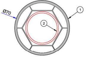
1. Açılı Köşe Dönüş Borusu P.A.070.5106.600.0.00.19 2. Destek Sacı (Ø42mm) 1,2mm - 34022 - 12502 1,5mm - 34022 - 15502 2 mm - 34022 - 20502
